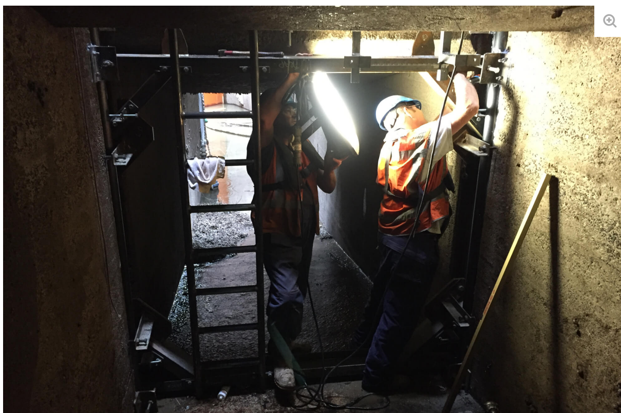
Het afstellen van geleidingen in het spoelrioolkanaal.
